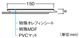
断面形状
