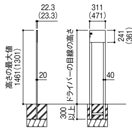
F33EX寸法図 (単位:mm) ※( )内はF48EX
